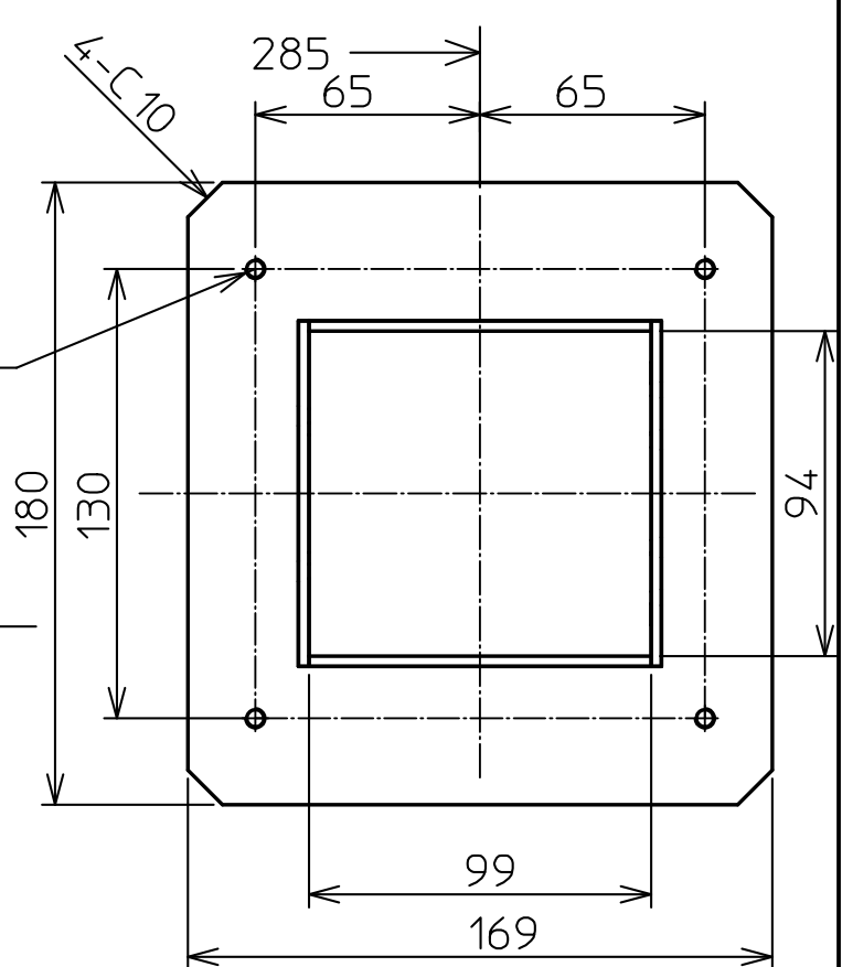
投入口詳細図
