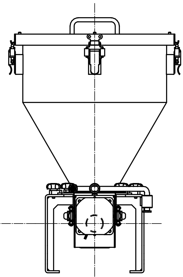
断面図 A-A
