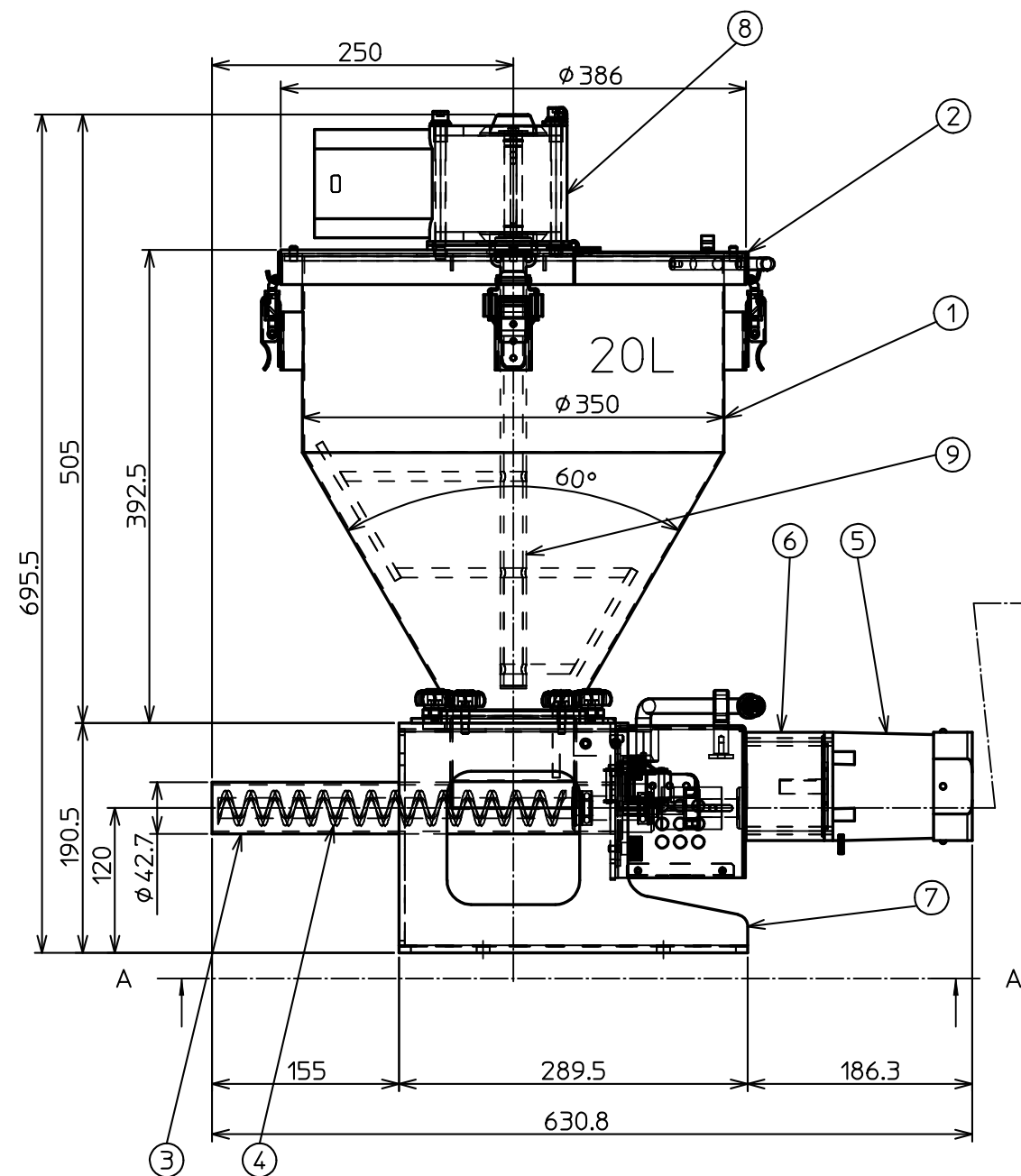
一般1 縮尺 1:7
