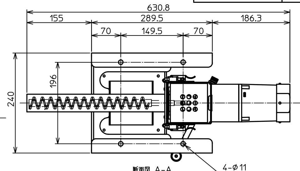
断面图 A-A
