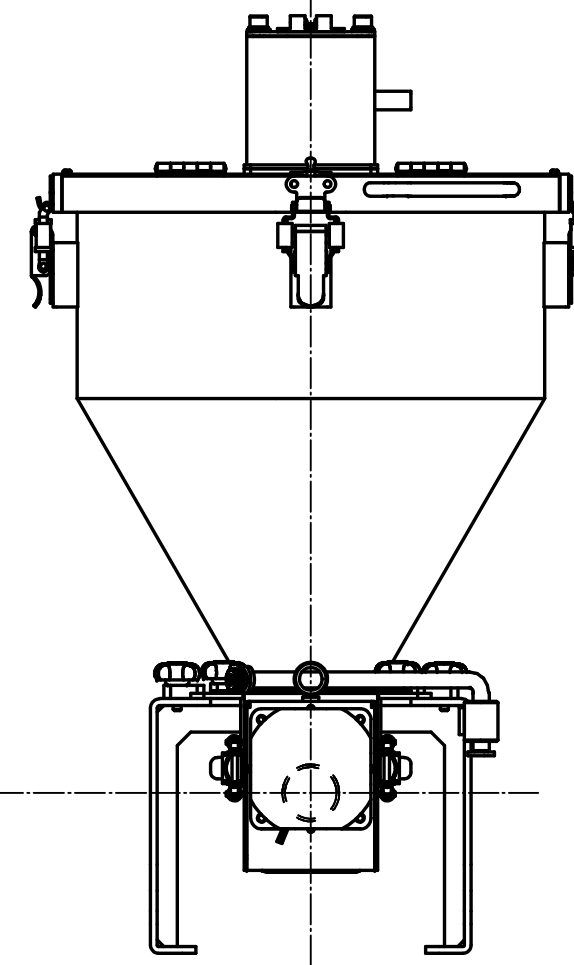
断面图 A-A
